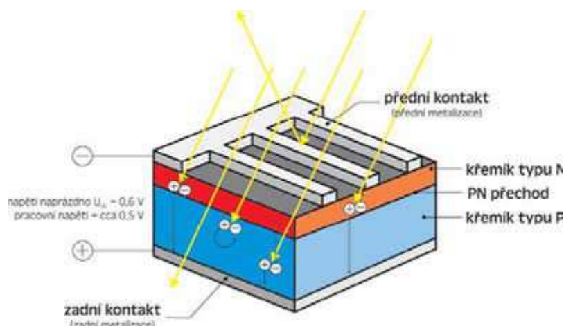
Princip činnosti solárního článku. © EkoWATT
