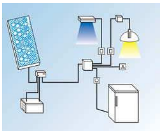
Schéma zapojení ostrovního systému. © EkoWATT
