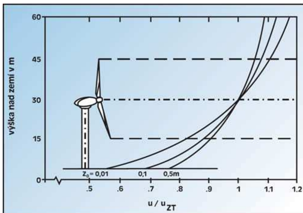
Schématizované vertikální profily rychlosti větru v přízemní vrstvě při různých parametrech drsnosti. Zdroj: časopis Větrná energie
