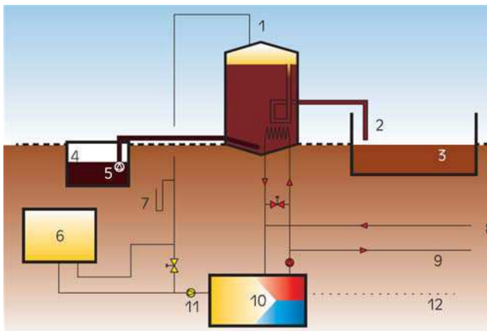
Schéma bioplynové stanice, kontinuální systém. © EkoWATT
